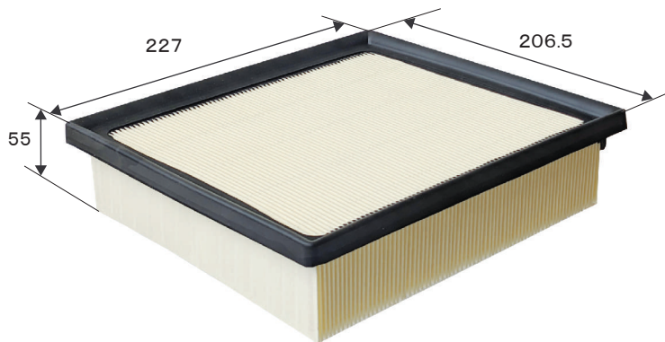
エレメント参考図
