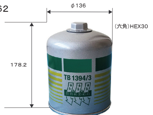
ネジ径 G1-1/4
